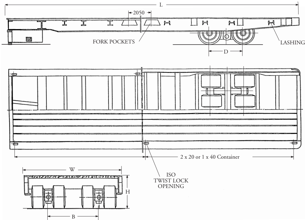
40' Rolltrailer
